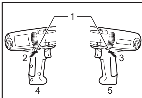
► 1. Palanca del conmutador de inversión de giro 2. Lado A 3. Lado B 4. En sentido de las manecillas del reloj 5. En sentido contrario a las manecillas del reloj
